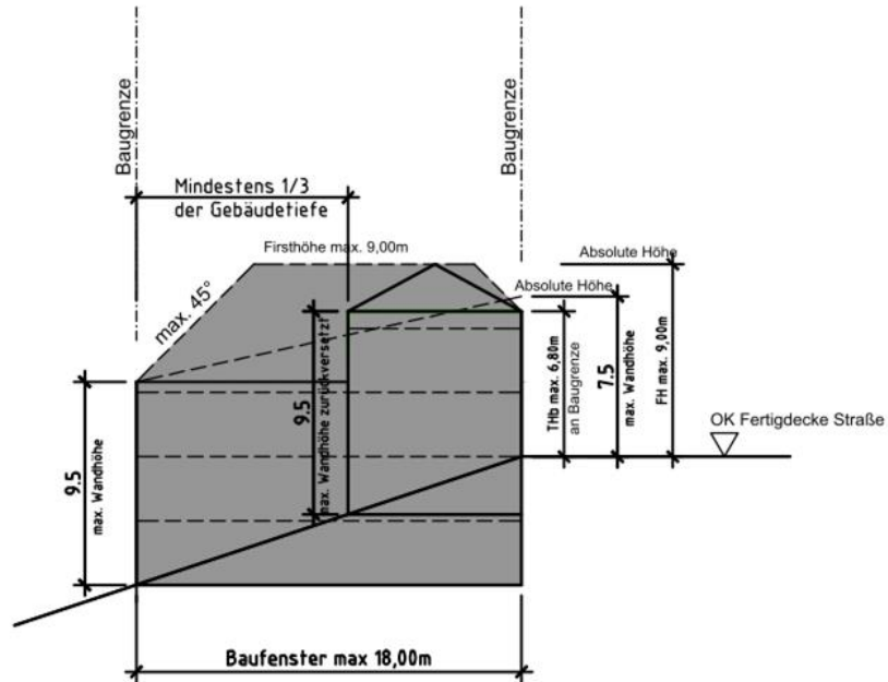
N1 - Allgem. Wohngebiet SYSTEMSCHNITT A-A
